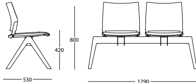
Panca due posti Two seats bench Bancada dos asientos
