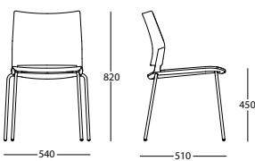
Quattro gambe Four legs frame Cuatro patas
