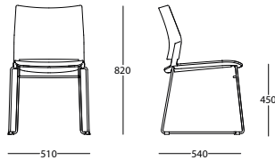
Fusto tondino Rod tube Base de varilla
