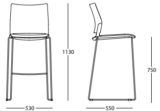
Sgabello Barstool Taburete
