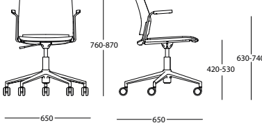
Base girevole con braccioli Swivel base with armrests Base giratoria con reposabrazos
