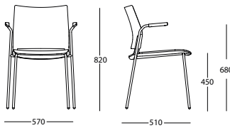
Quattro gambe con braccioli Four legs frame with armrests Cuatro patas con reposabrazos
