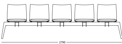
Panca cinque posti Five seats bench Bancada cinco asientos
