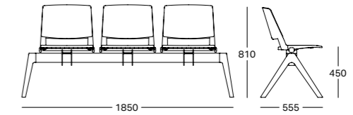
Panca 3 posti con gamba GP04 3 seater bench with GP04 leg Banco de 3 plazas con pata GP04
