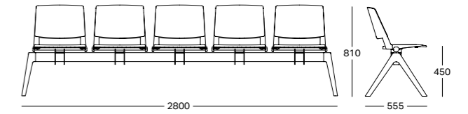
Panca 5 posti con gamba GP04 5 seater bench with GP04 leg Banco de 5 plazas con pata GP04
